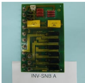
品番 MI-004 基板名 INV-SNBA 取付部 カゴ上 用途 ドアマシン用トランジスタのスナバ回路
