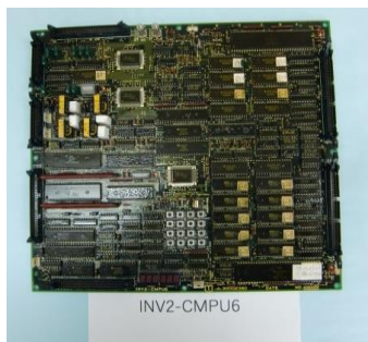
品番 MI-001 日立 B89インバーター(1994.9) 基板名 INV2-CMPU6 取付部 制御盤 用途 主・従マイコン基板 新品単価 ¥470,000
