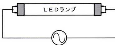
1灯式配線図
