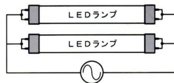
2灯式配線図
